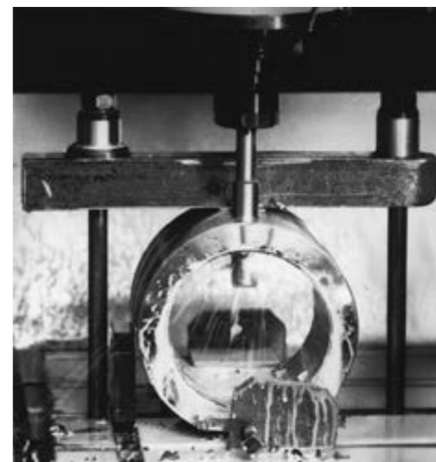
Lamage en tirant avec arrosage central.
