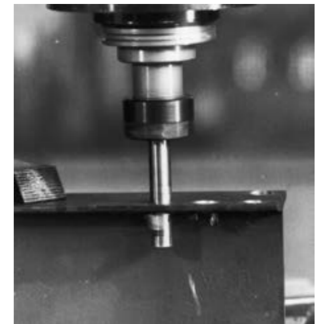
Lamage en tirant avec rayon.
